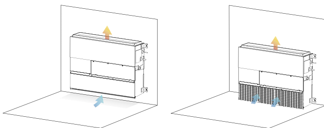
Bodenabsaugung/Wandbefestigung
